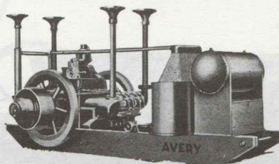
Avery Skid Motor
