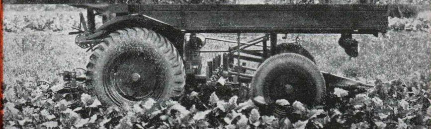
Das zwischen den Achsen eingebaute, leicht ein- und aushebbare und beim Arbeiten voll zu überblickende Hackgerät ist ein ideales Werkzeug für alle Hack- und Saatzarbeiten. Der FARMAX hilft dem Bauern zu intensiver Bodenkultur.
